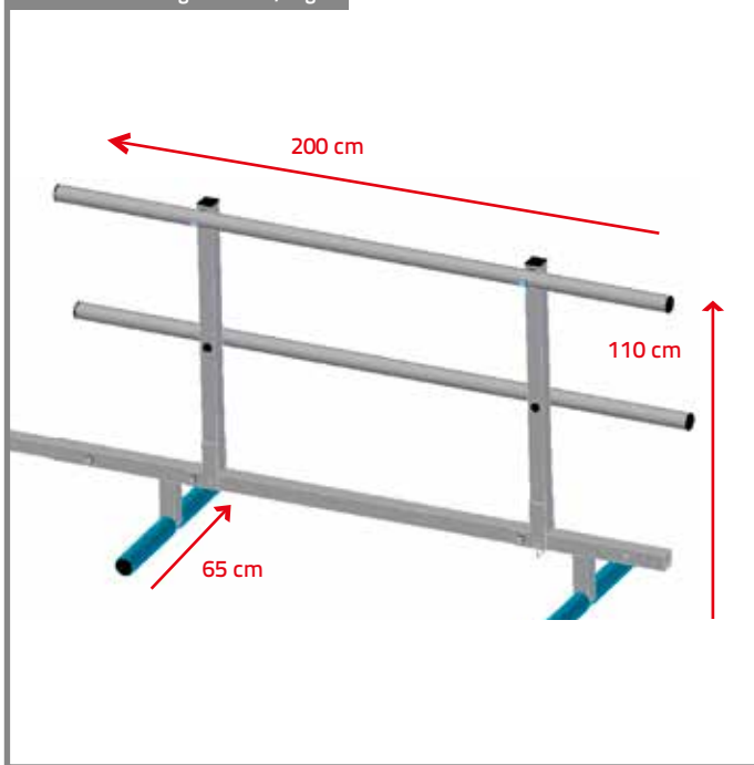
2 m Hekwerk / gewicht 12,4 kg
